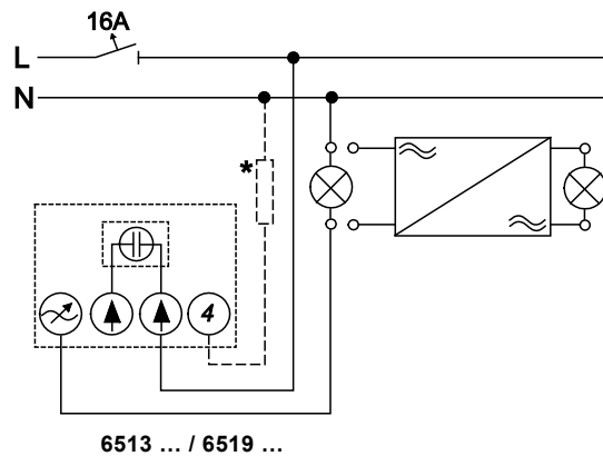
图 4: 使用电压传感器的调光器运行
