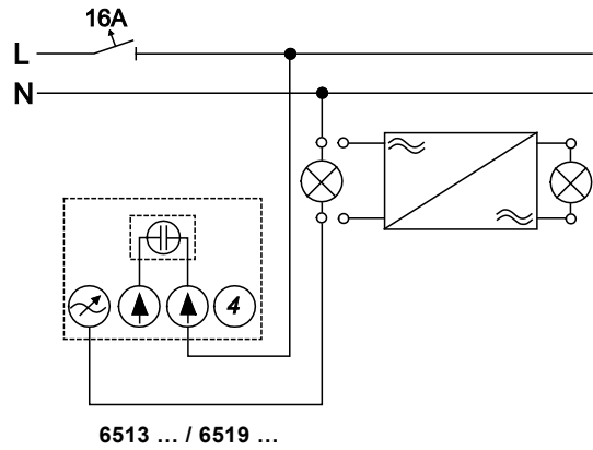
图 2: 调光器运行
