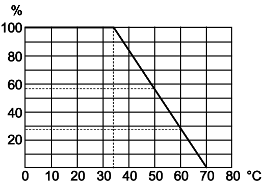
图 1：降低额定值
