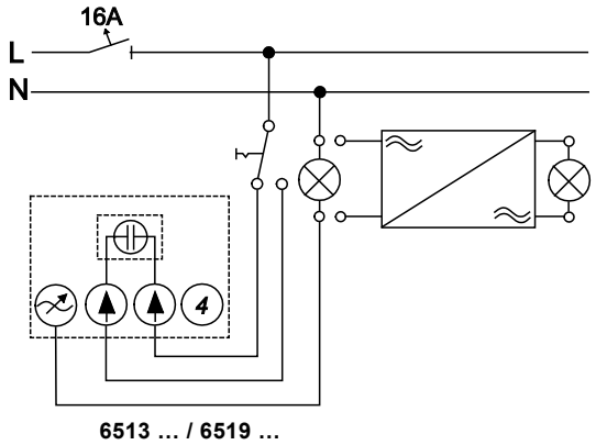
图 3: 交流电路中的调光器
